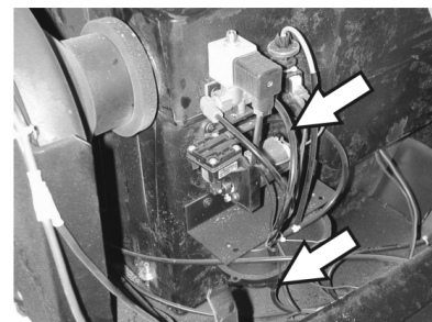
Alipainepumpun ja alipainerasian letkuliitäntä (varaaja)
