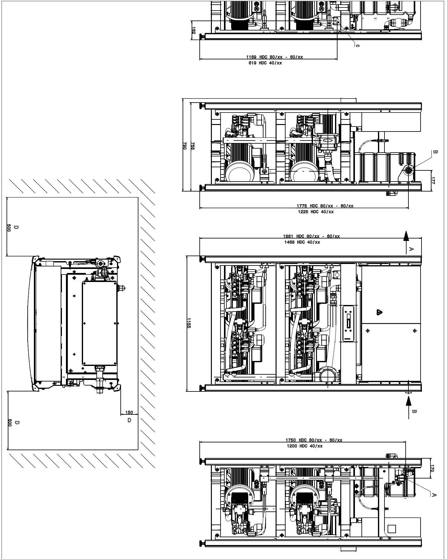
A HDC 80/16 H ábrázolása burkolólemezek nélkül
